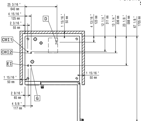
Felülnézet
